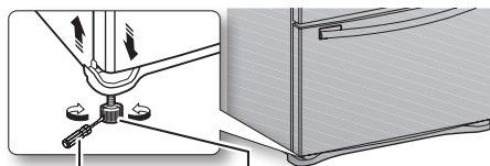
Desarmador de punta chata (-) Palanca de control chata (-)
