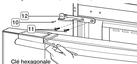
Clé hexagonale
