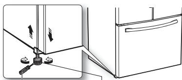
tournevis à lame plate (-) Molette
