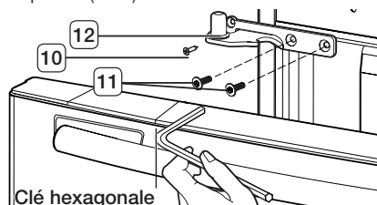
Clé hexagonale
